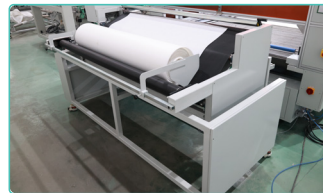
自动送料机
